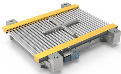
PALLET ROTATOR
